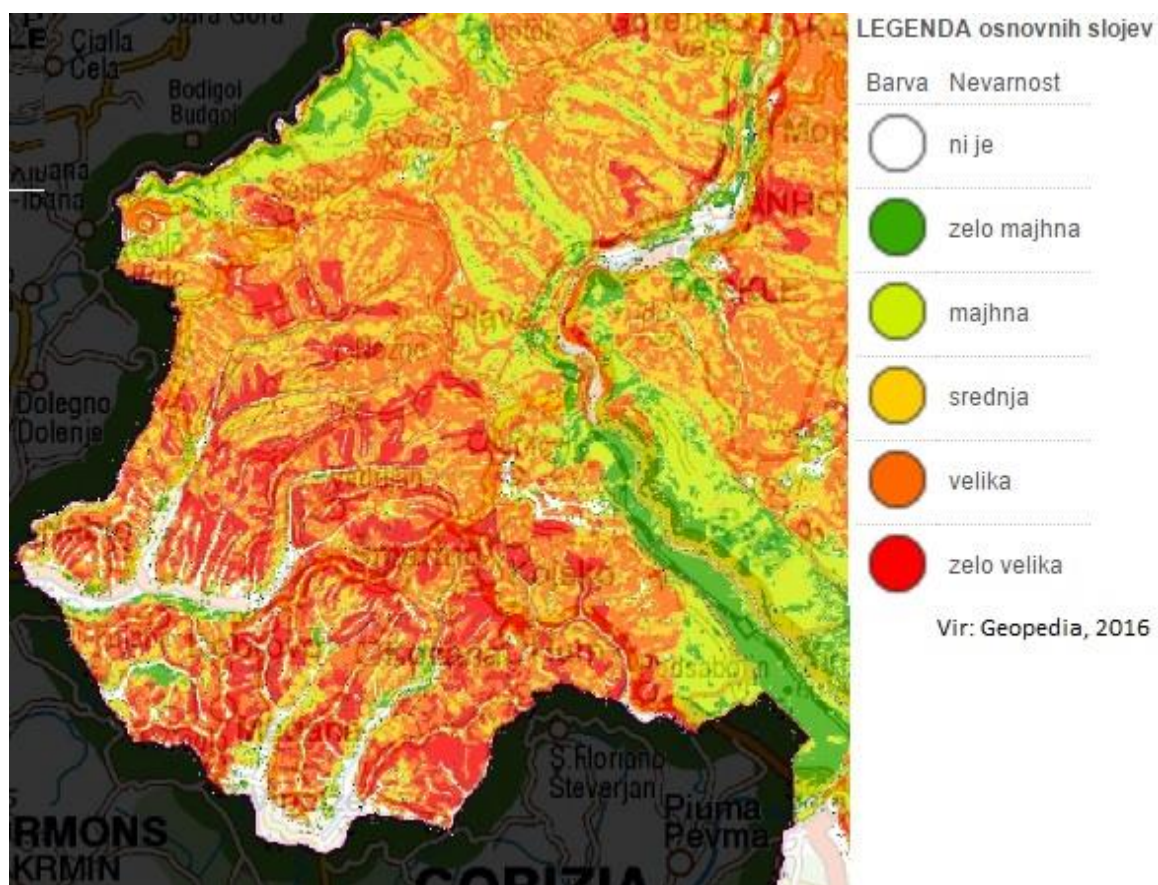
Slika 1: Verjetnost pojavljanja plazov na območju občine Brda
